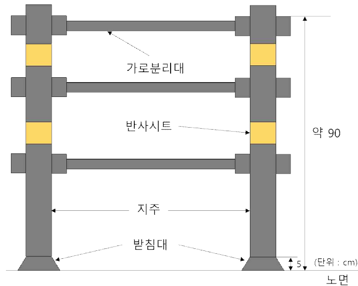
<그림 1> 무단횡단 금지시설의 형상(예시)
